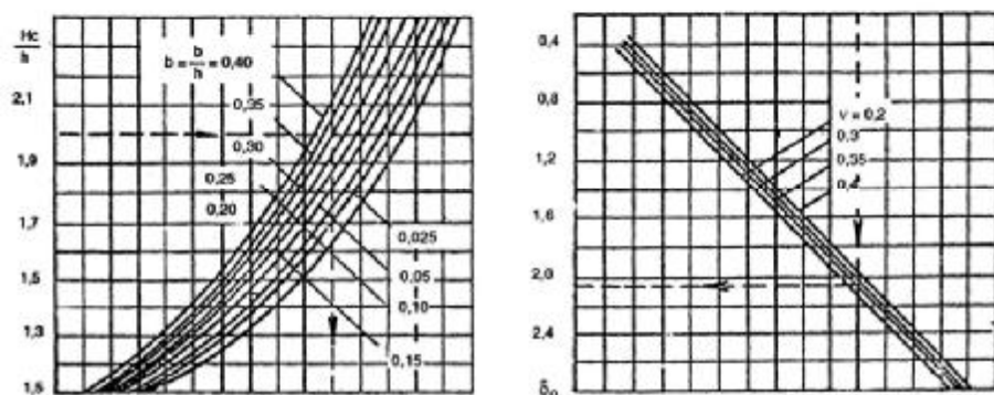
Hình H.5 : Biểu đồ dùng xác định \delta_0 .
