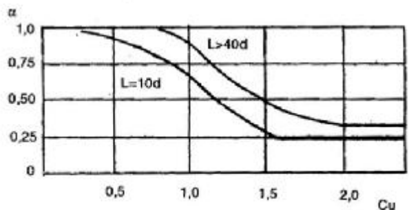
Hình B1: Quan hệ \alpha - c_u
