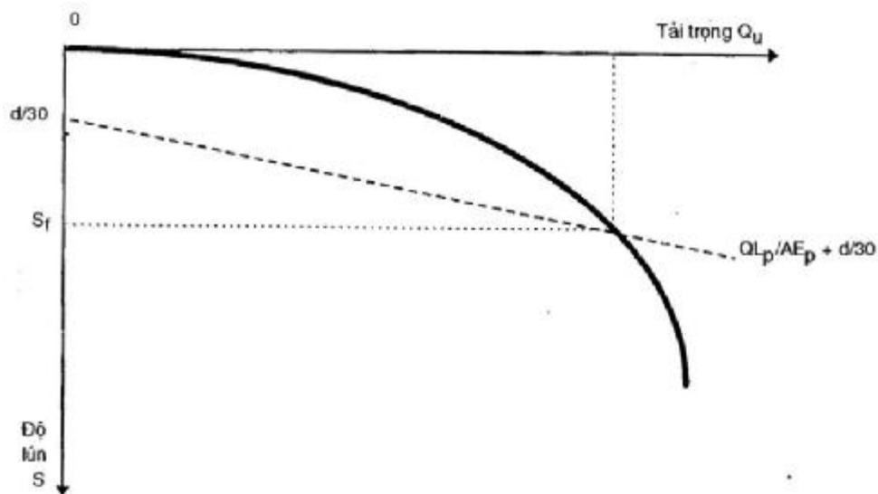
Hình E.2 : Phương pháp xác định Q_u theo công thức (E4)
