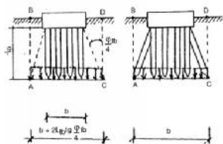
Hình H.1 : Kích thước móng quy ước xác định theo cách 1 o .
