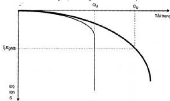
Hình E.1 : Phương pháp xác định Q_u theo công thức (E.3)
