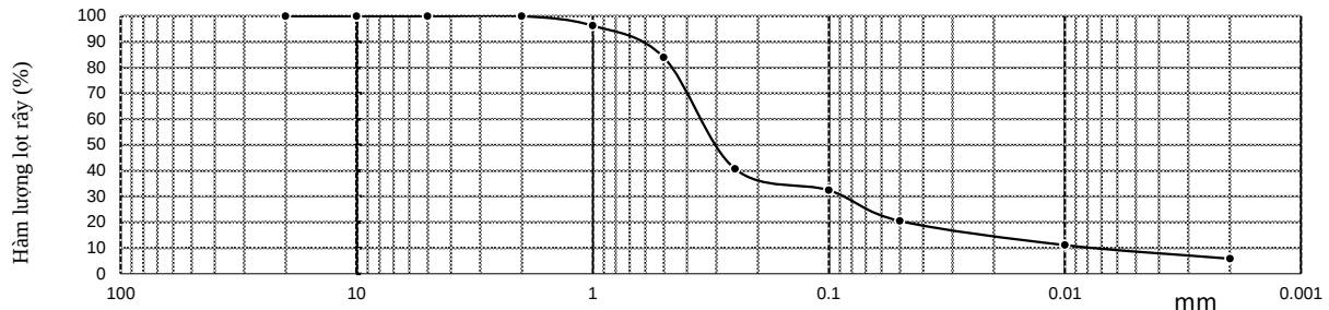
Đồ thị thí nghiệm thành phần hạt
