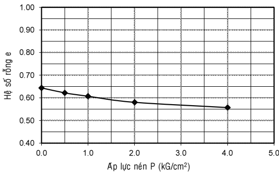
Đồ thị thí nghiệm nén lún
