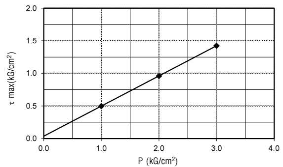
Đồ thị thí nghiệm cắt phẳng
